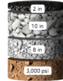
Unstabilized 111,200 ESALs
