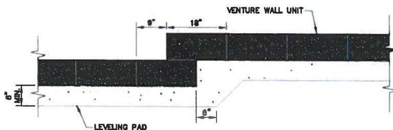
« LEVELING PAD DETAIL »
