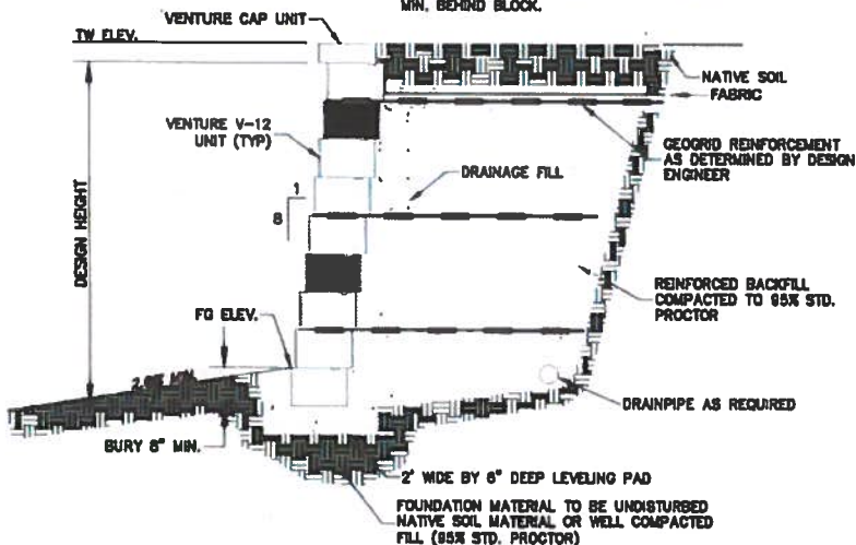
« TYPICAL RETAINING WALL SECTION »
