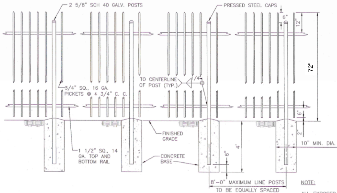
ORNAMENTAL IRON FENCE DETAIL N.T.S.
