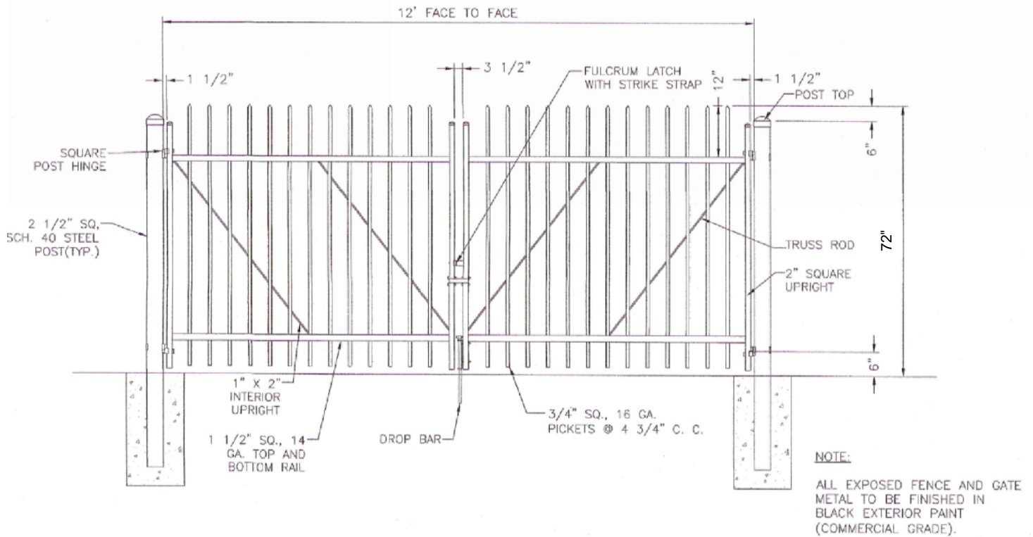
ORNAMENTAL IRON GATE DETAIL N.T.S.
